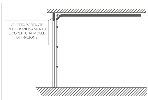
SEZIONE LATERALE - MONTAGGIO IN LUCE
