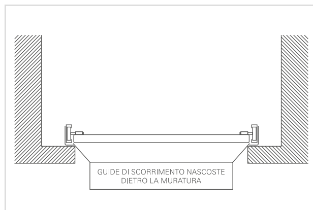
VISTA IN PIANTA - MONTAGGIO OLTRE LUCE
