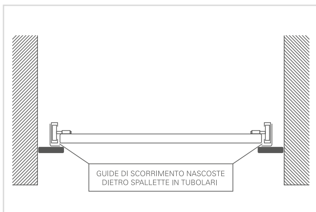
VISTA IN PIANTA - MONTAGGIO IN LUCE
