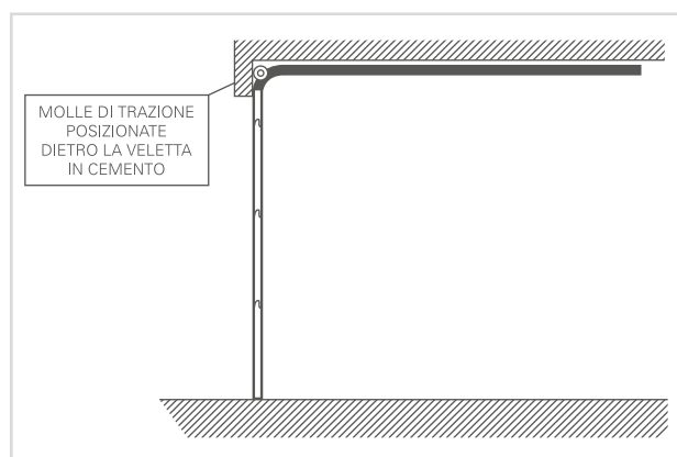
SEZIONE LATERALE - MONTAGGIO OLTRE LUCE
